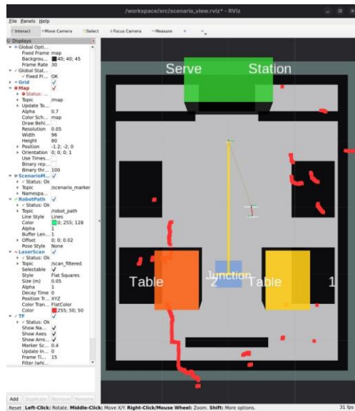
รูปที่ 45 แผนที่ของหุ่นยนต์ระหว่างเดินไปยังจุด Junction โปรแกรม Rviz2
