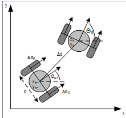
รูปที่ 7 การคำนวณตำแหน่งของหุ่นยนต์บนแผนที่โดยหลักการ Odometry โดยจะใช้ค่า รัศมีล้อ ระยะห่างระหว่างล้อ ระยะทางที่ล้อขยับแต่ละข้าง โดยได้ผลลัพธ์ออกมาคือตำแหน่ง และมุมของหุ่นยนต์ (ที่มา: https://hackaday.io/project/158496-imcoders/log/147068-robot-odometry )
