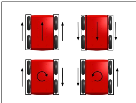
รูปที่ 6 ลักษณะการขับเคลื่อนด้วยวิธี Differential Drive โดยการสั่งให้ล้อไปทางเดียวกันคือการไปข้างหน้า หรือไปหลัง ส่วนการสั่งให้ล้อขับเคลื่อนตรงข้ามกันด้วยความเร็วเท่ากันจะทำให้หุ่นยนต์หมุนรอบตัวเอง (ที่มา: https://existentialrobotics.org/RobotProvingGrounds/algorithms/control/content/diffy_drive/ )
