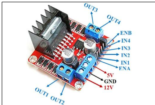
รูปที่ 4 มอดูล L298N H-Bridge
