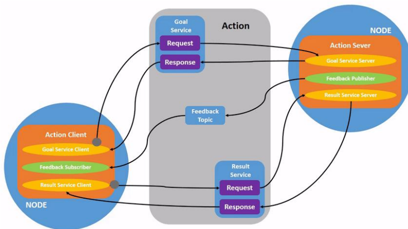
รูปที่ 12 แผนภาพการทำงานของ ROS Action: Client ส่งเป้าหมายให้ Server, รับความคืบหน้าผ่าน Topic และรับผลลัพธ์เมื่อทำงานเสร็จ (ที่มา: https://docs.ros.org/en/dashing/Tutorials/Understanding-ROS2-Actions.html )
